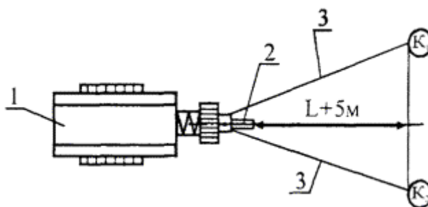
K_1, K_2 - рабочие места копровщиков, L - длина сваи 1 - сваебойная установка, 2 - свая, 3 - оттяжка.
