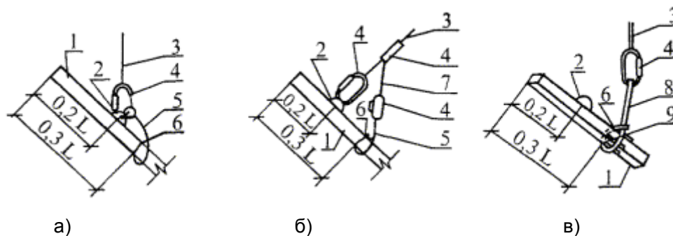
Рисунок 3 - Строповка свай длиной до 6 - 8 м (а, б) и более 6 - 8 м (в) при подъеме на копер
