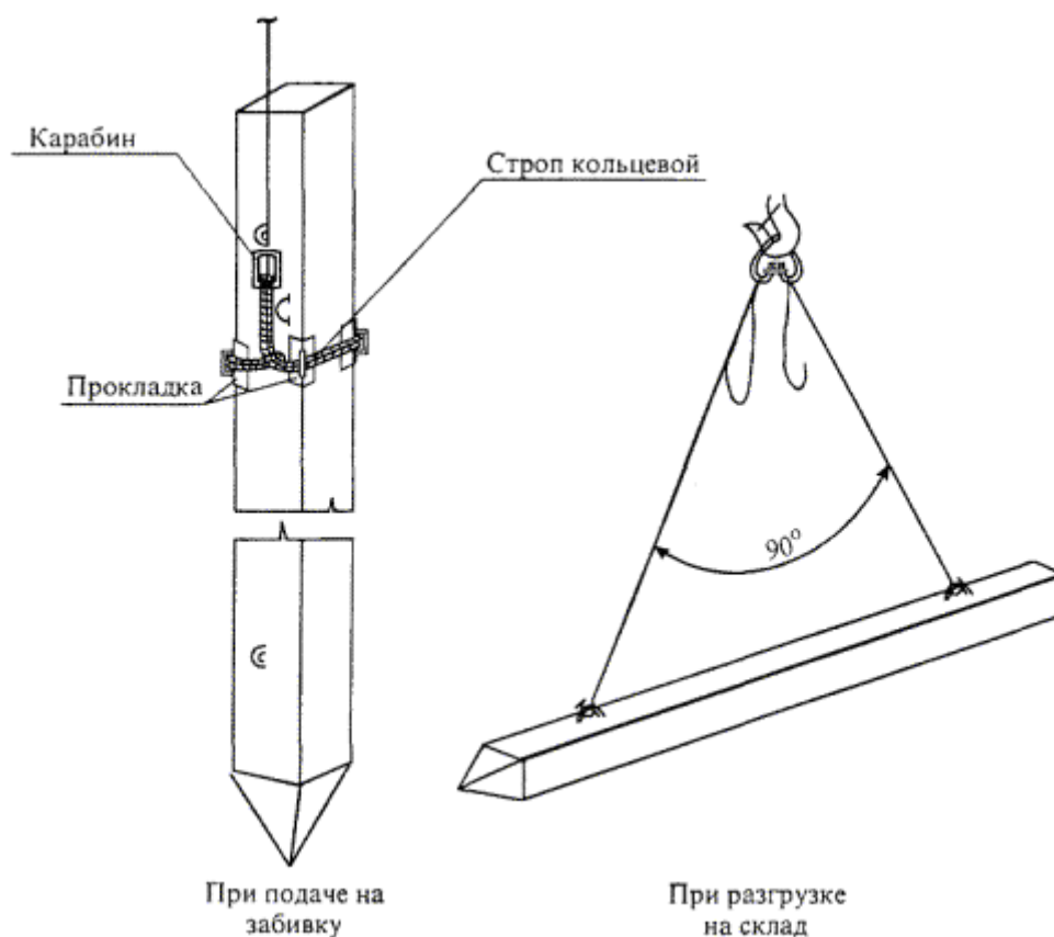
Рисунок 9 - Схемы строповок свай
