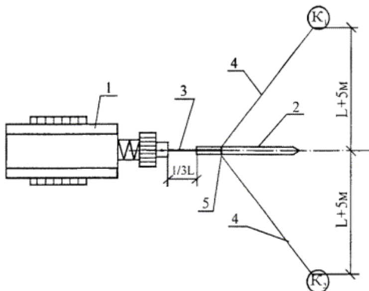
K_1, K_2 - рабочие места копровщиков, L - длина сваи 1 - копровая установка, 2 - свая, 3 - кольцевой строп, 4 - оттяжки (пеньковый канат \varnothing 16 - 18 мм), 5 - хомут для закрепления оттяжек
