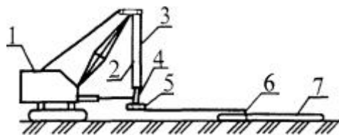
Рисунок 1 - Схема подтаскивания сваи:
