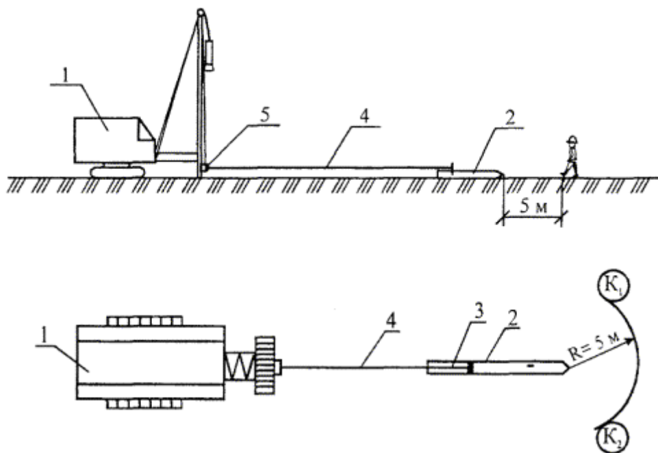
Рисунок 2 - Схема организации рабочего места при подтаскивании свай.
